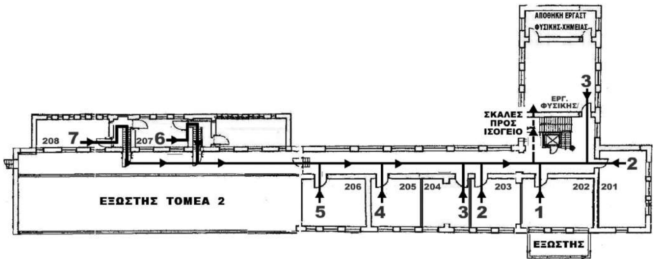
Κάτοψη Πίσω Πτέρυγας
